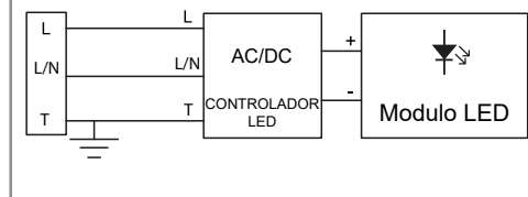
CARACTERÍSTICAS DEL CONTROLADOR LED X6-105M150
