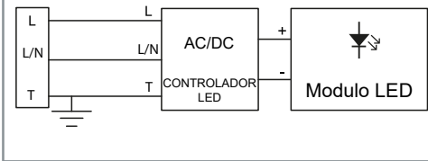
CARACTERÍSTICAS DEL CONTROLADOR LED X6-200M286
