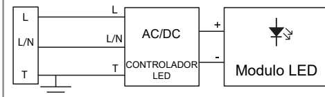
CARACTERÍSTICAS DEL CONTROLADOR LED DL-50W-V72A-MXG
