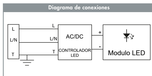
CARACTERÍSTICAS DEL CONTROLADOR LED X6-200M286
